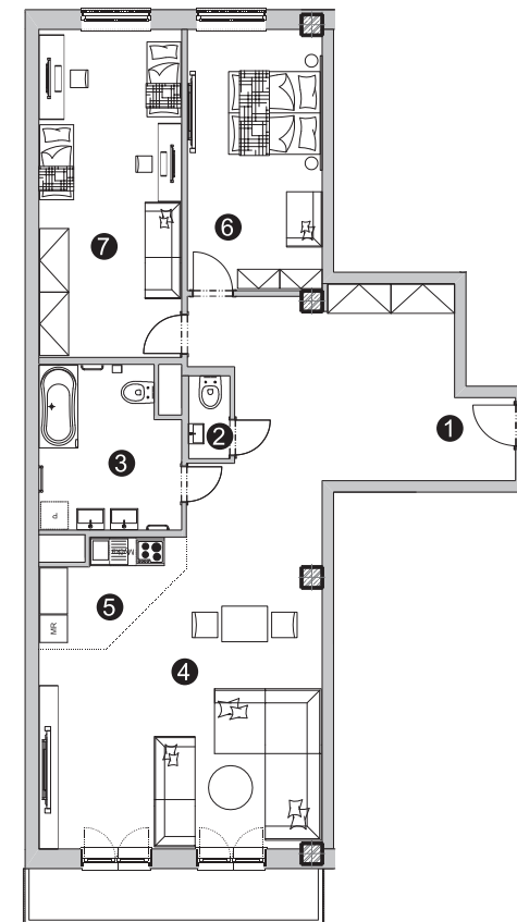
Půdorys podlaží | Floor plan
